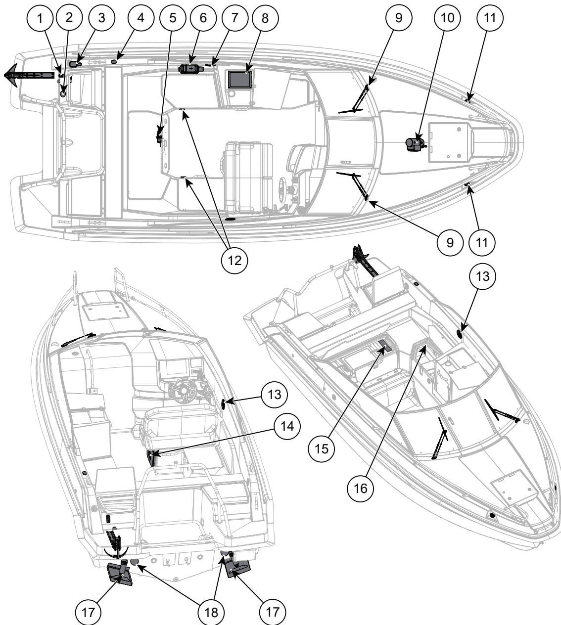
Figure 8.2 Yamarin 67 DC - Équipement électrique
