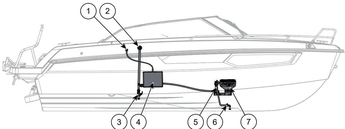
Figure 11.1 Yamarin 67 DC - Système septique
