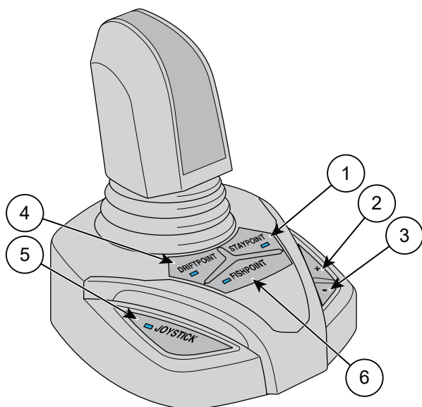
Figure 5.4 Joystick et boutons de fonction
