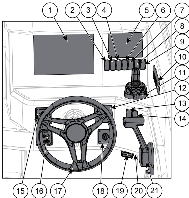
Figure 5.1 Yamarin 67 DC - Commandes du poste de barre
