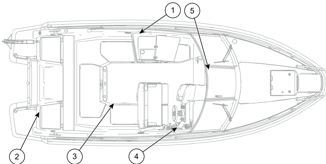
Figure 2.1 Yamarin 67 DC - Étiquettes de sécurité
