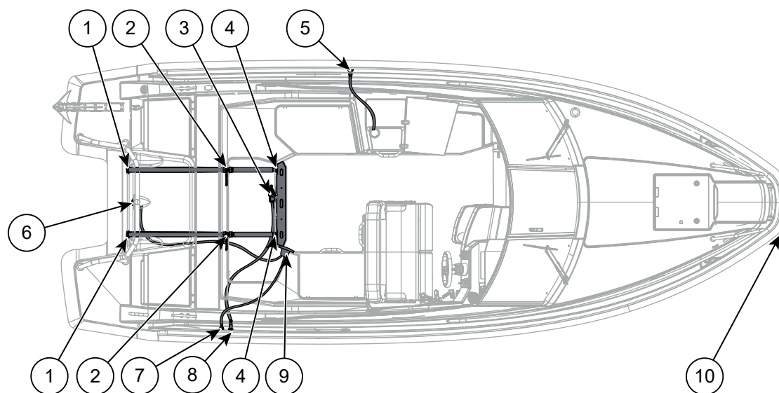
Figure 9.1 Yamarin 67 DC - Pompes et vidange de cale
