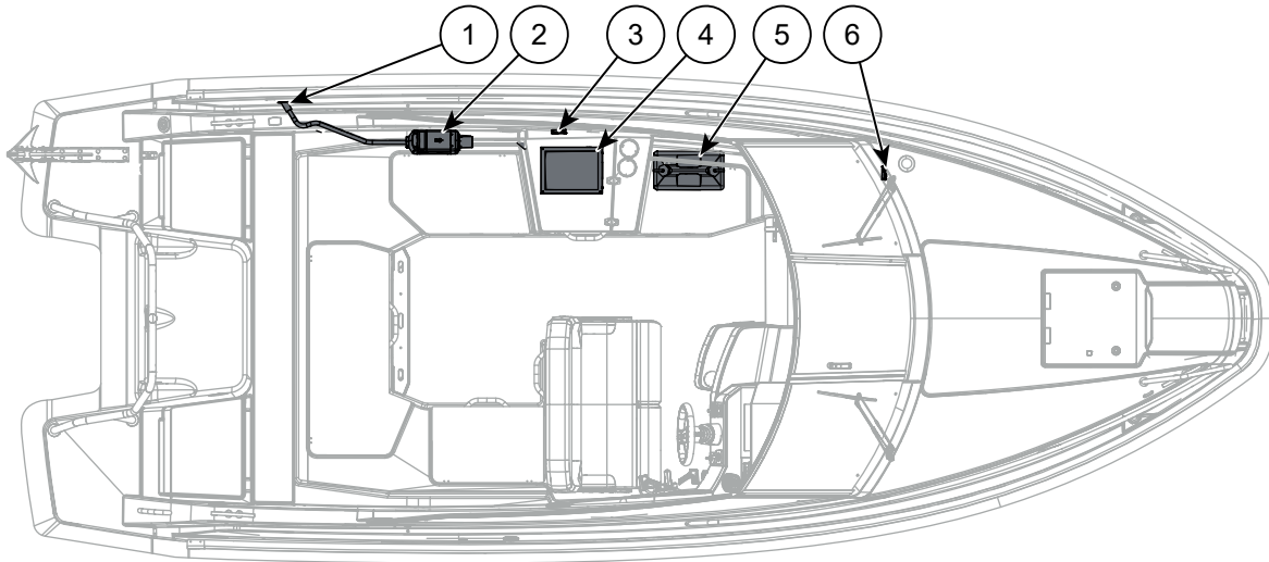
Figure 6.2 Yamarin 67 DC - Équipement alimenté en carburant
