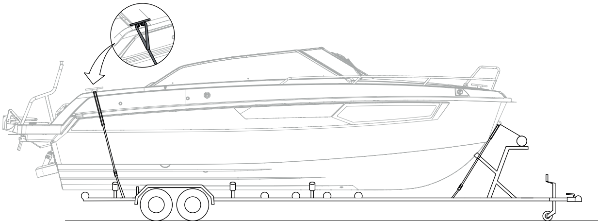
Figure 13.1 Yamarin 67 DC - Transport sur remorque
