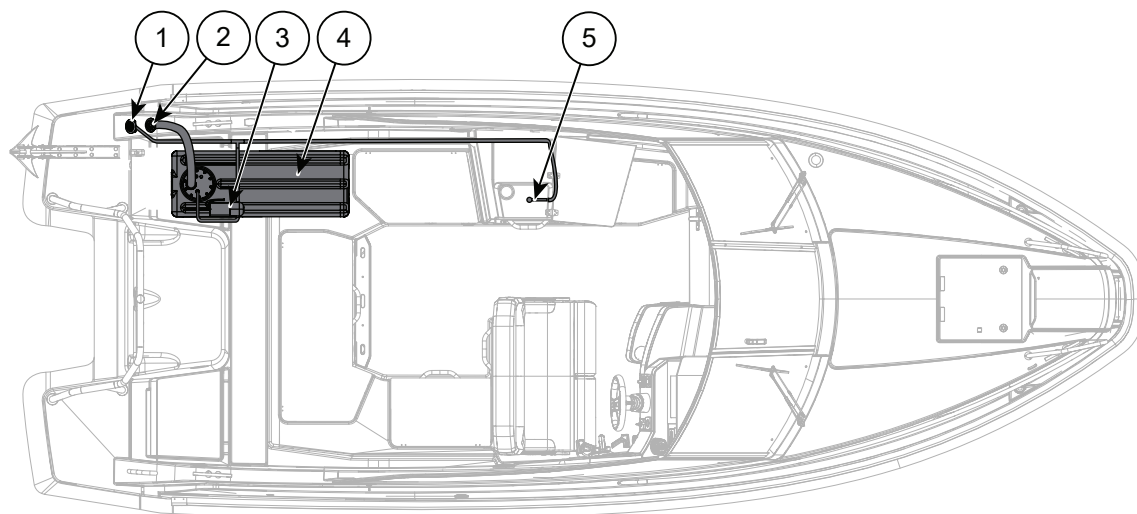
Figure 10.1 Yamarin 67 DC - Système d'eau douce
