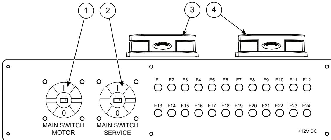
Figure 8.1 Yamarin 67 DC - Interrupteurs principaux et panneau de fusibles
